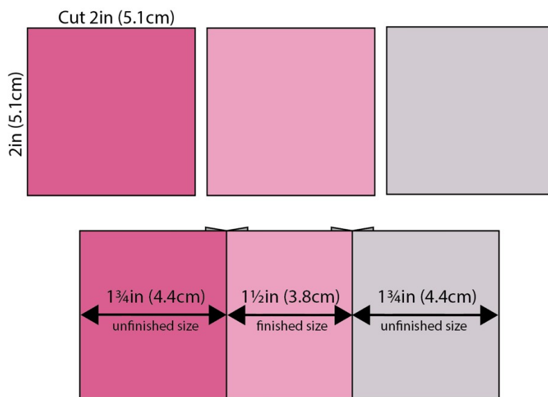
Fig. K Coutures précises
